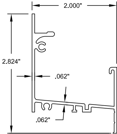
2 FRAME SILL 6063-T6 ALUMINUM
